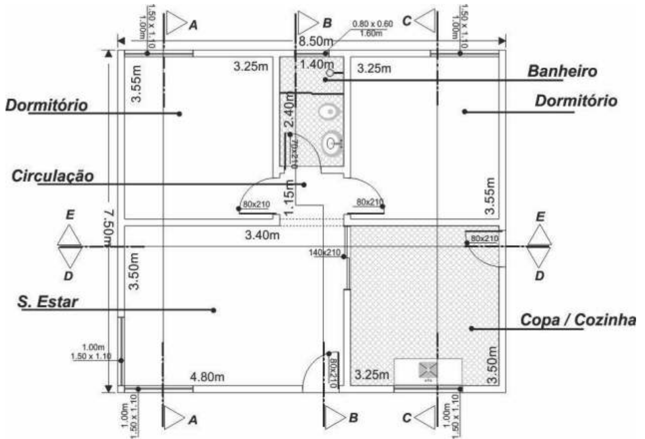
Planta Baixa - Técnica
