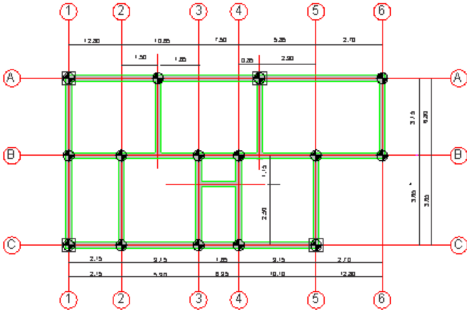
PLANTA LOCAÇÃO - EIXOS E FUNDAÇÃO
