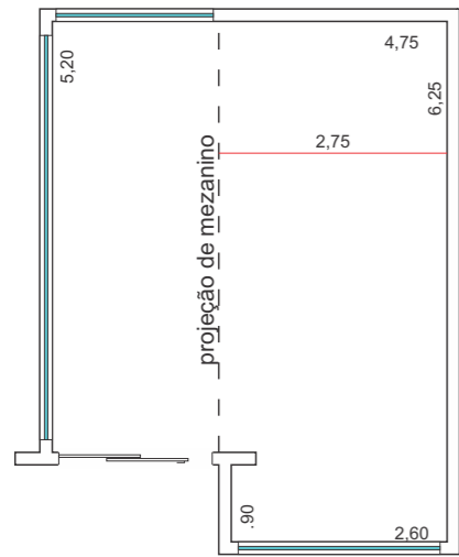
Planta baixa loja shopping pé direito = 4,90m alt. do mezanino = 2,5m
