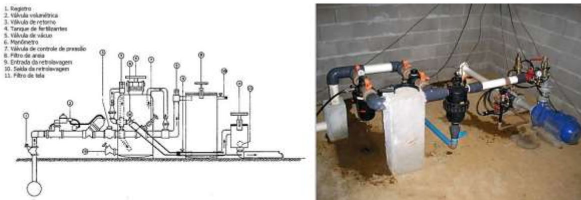
Figura 123: Esquema de cabeçal de controle para irrigação localizada (esquerda) e exemplo de um cabeçal montado em propriedade rural (direita) (Fonte: ANTUNES, 2016).
