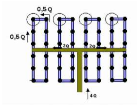
Figura 75: Diagrama do sistema de irrigação com distribuição por malha (Fonte: Adaptado de DRUMOND & FERNANDES, 2001).
